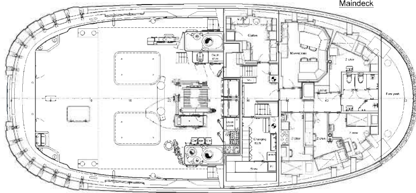
Maindeck
